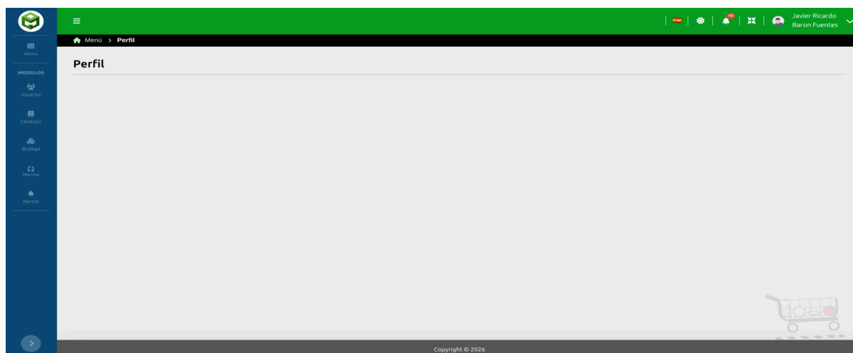
Figura 16: Opción “perfil”.
