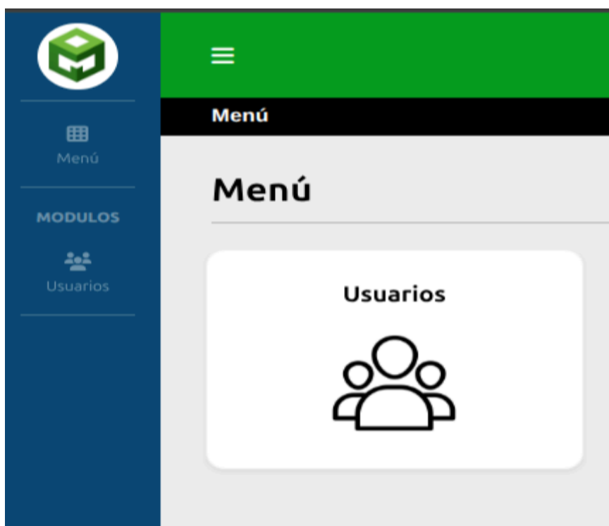
Figura 24: Módulo usuarios.
